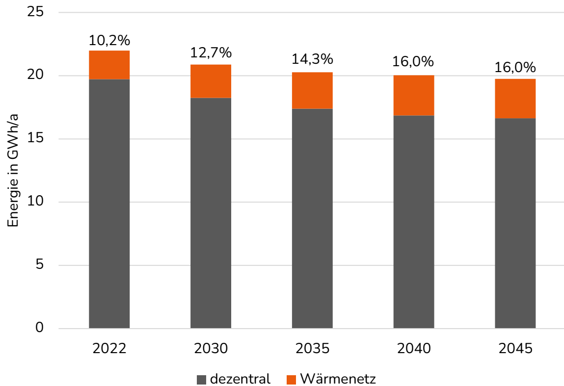
Abbildung 48: Anteil leitungsgebundener Wärme am gesamten Wärmeverbrauch in den Stützjahren (Veröffentlichung nach WPG, Anlage 2, III.)
