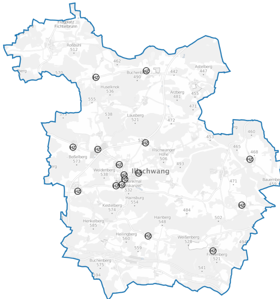
Abbildung 12: Hackschnitzelheizungen zur Versorgung privater Wärmenetze im Gemeindebereich
